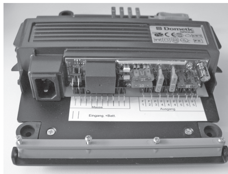
Op de foto is het apparaat zonder afdekkap te zien.
