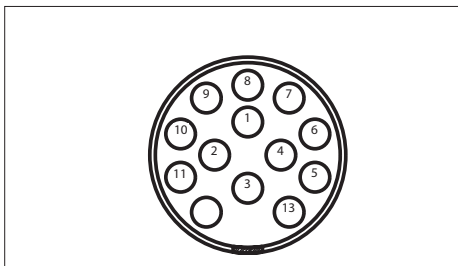
Contactdoos Jäger 13-polig
