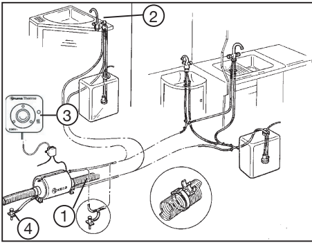
Schema van de watervoorziening
